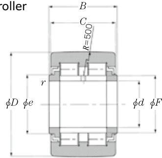
NUTW2 type
